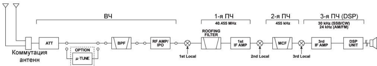
Блок-схема приемника
