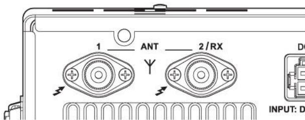
Разъемы антенн на задней панели трансивера
